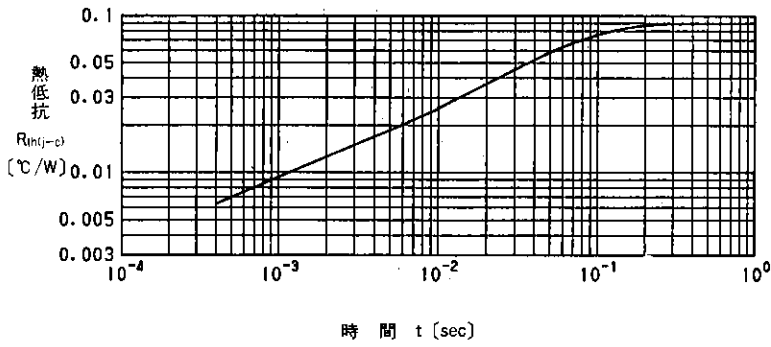
時間 t (sec) 過渡熱抵抗(トランジスタ)特性 Transient Thermal Resistance (Transistor)
