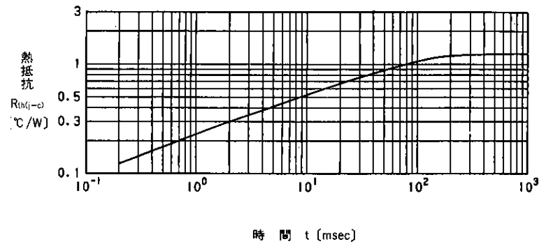
時間 t (msec) 過渡熱抵抗(ツェナーダイオード)特性 Transient Thermal Resistance (Zener Diode)
