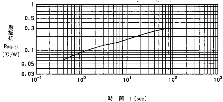
時間 t (sec) 過渡熱抵抗(ダイオード)特性 Transient Thermal Resistance (F.R.D)
