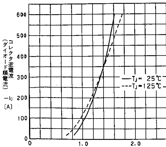
エミッタ・コレクタ間電圧 V_{ce0} (V) (ダイオード順電圧) 高速フリーホイーリングダイオード順電圧特性 Forward Voltage of Free Wheeling Diode
