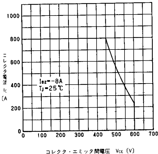
安全動作領域(逆バイアス) Reverse Bias Safe Operating Area
