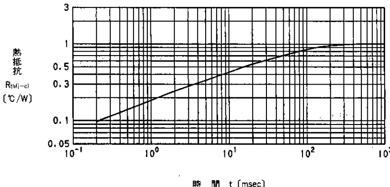
時間 t (msec) 過渡熱抵抗(ツェナーダイオード)特性 Transient Thermal Resistance (Zener Diode)
