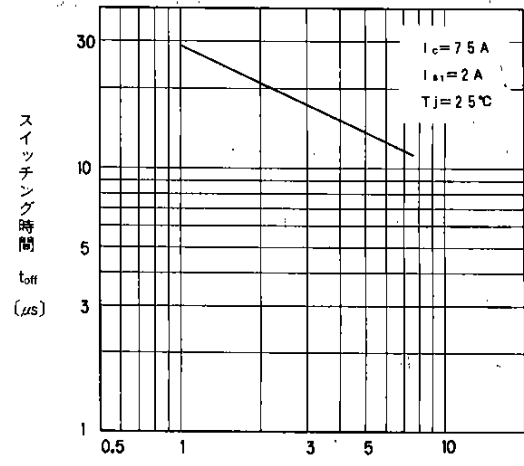
ベース電流 -I_{e2} [A] スイッチング時間-ベース電流特性 Switching Time
