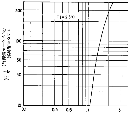
コレクタ逆電流 (ダイオード順電流) -I_c [A] エミッタ・コレクタ間電圧 V_{eco} [V] (ダイオード順電圧) 高速フリーホイリングダイオード順電圧 Forward Voltage of Free Wheeling Diode
