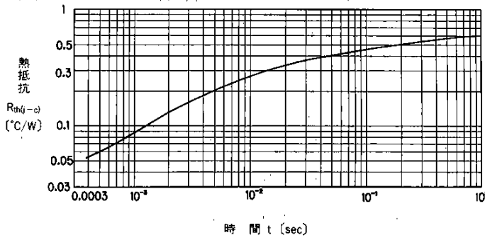
熱抵抗 R_{th(j-d)} [°C/W] 過渡熱抵抗(ダイオード)特性 Transient Thermal Resistance (Diode)
