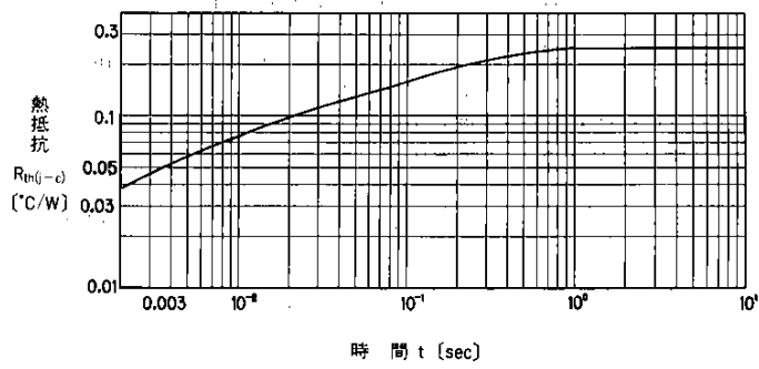
熱抵抗 R_{th(j-c)} [°C/W] 過渡熱抵抗(トランジスタ)特性 Transient Thermal Resistance (Transistor)
