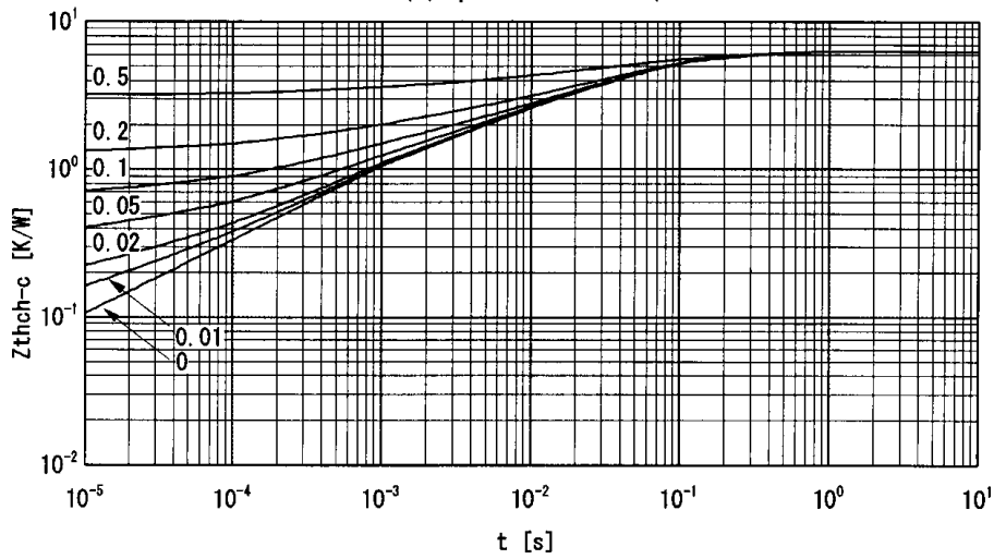
Transient thermal impedande Z_{thch}=f(t) parameter: D=t/T
