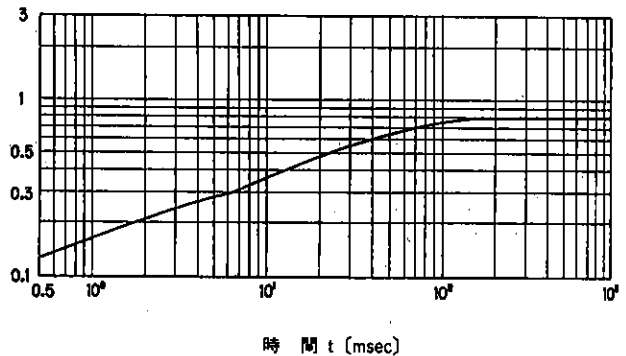
過渡熱抵抗(ダイオード)特性 Transient Thermal Resistance (Diode)
