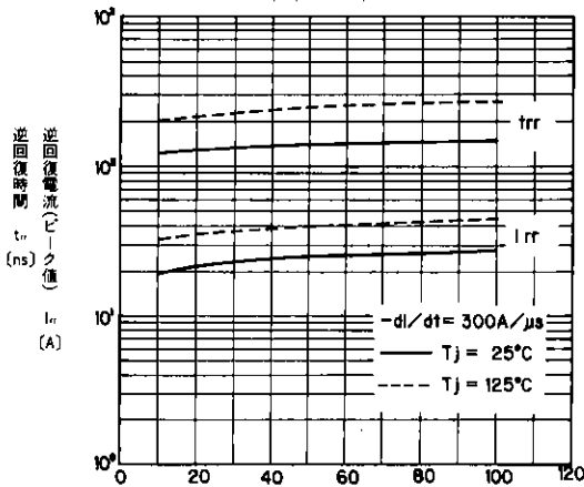
ダイオード順電流 I_r (A) trr, Irr-If特性 Trr, Irr-If
