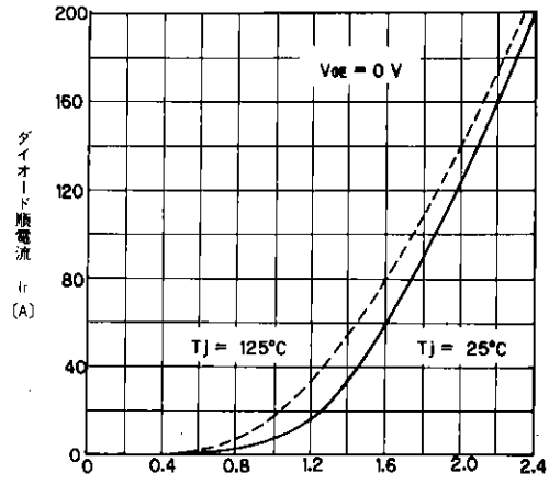
ダイオード順電圧 V_{fr} (V) 高速フリーホイールダイオード順電圧特性 Forward Voltage of Free Wheel Diode
