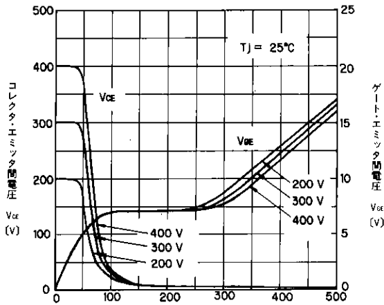
充電電荷量 Q_e (nC) ダイナミック入力特性 Dynamic Input Characteristic
