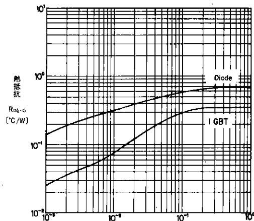
パルス幅 P_w (sec) 過渡熱抵抗 Transient Thermal Resistance
