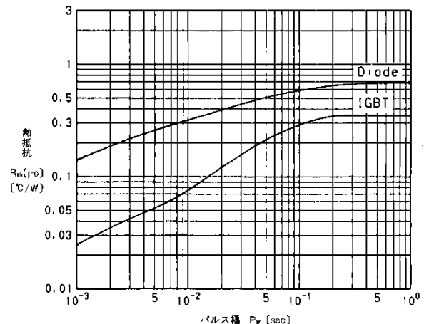
過渡熱抵抗特性 Transient Thermal Resistance
