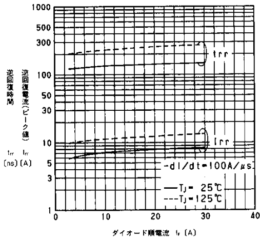
T_{rr} , I_{tr} - I_r 特性 T_{rr} , I_{tr} - I_r
