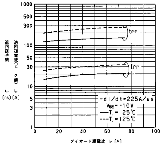
ダイオード順電流 I_{rr} (A) T_{rr} , I_{rr} - I_r 特性 T_{rr} , I_{rr} - I_r
