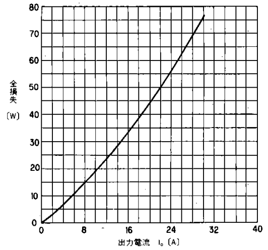
出力電流 - 損失 Output Current - Total Loss
