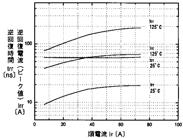
Trr, Irr-If特性 <INV部> Trr, Irr-If <INV>
