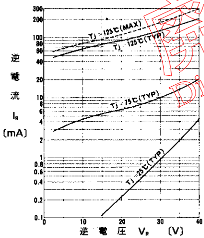
逆特性
