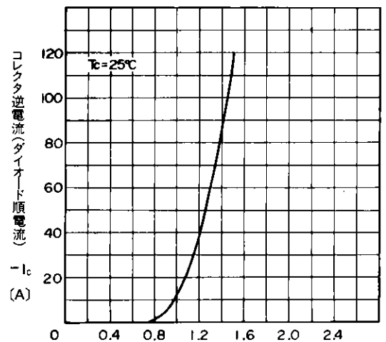
高速フリーホイリングダイオード順特性 Forward Voltage of Free Wheeling Diode
