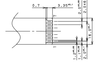
コネクタ接続部 (導通面) Connector (Conductive side)
