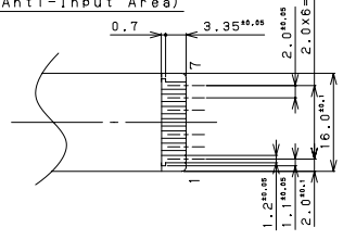
コネクタ接続部 (導通面) Connector (Conductive side)
